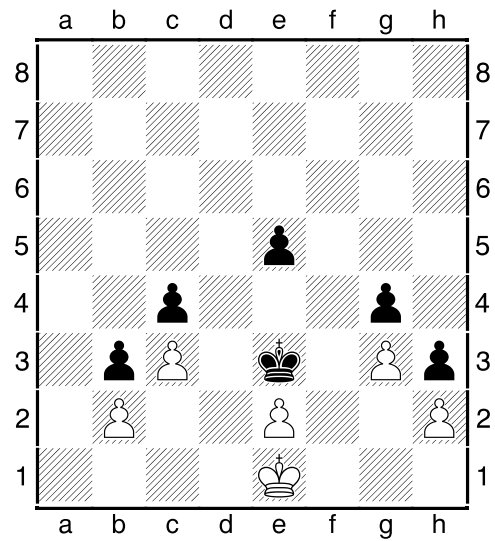
10 (remis)
